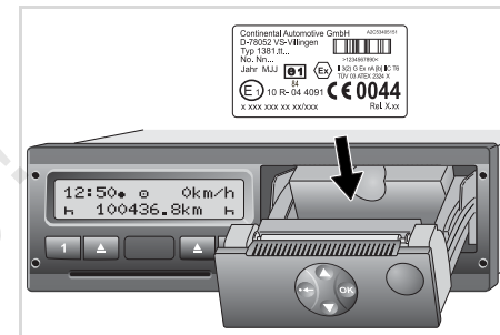
Típustábla
